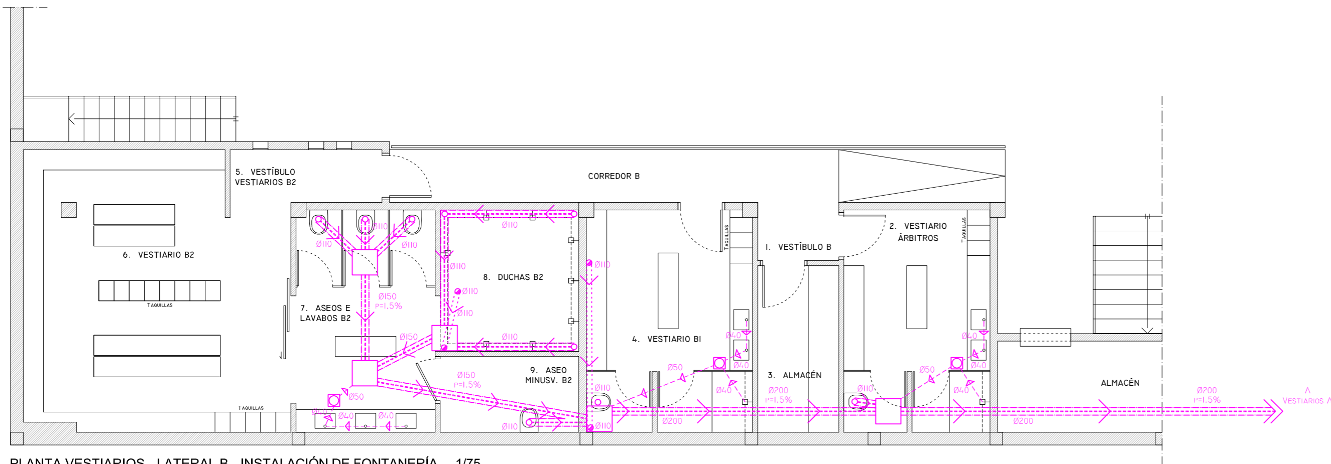
PLANTA VESTIARIOS - LATERAL B - INSTALACIÓN DE FONTANERÍA 1/75
