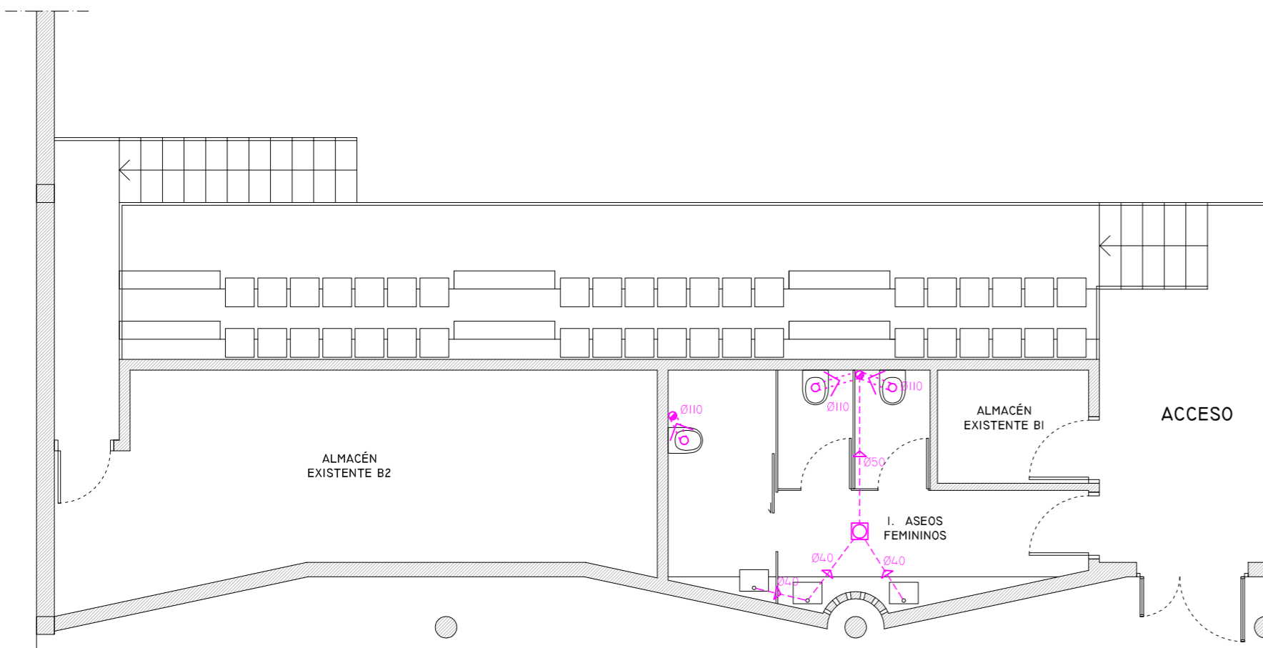
PLANTA ASEOS - LATERAL B - INSTALACIÓN DE FONTANERÍA 1/75
