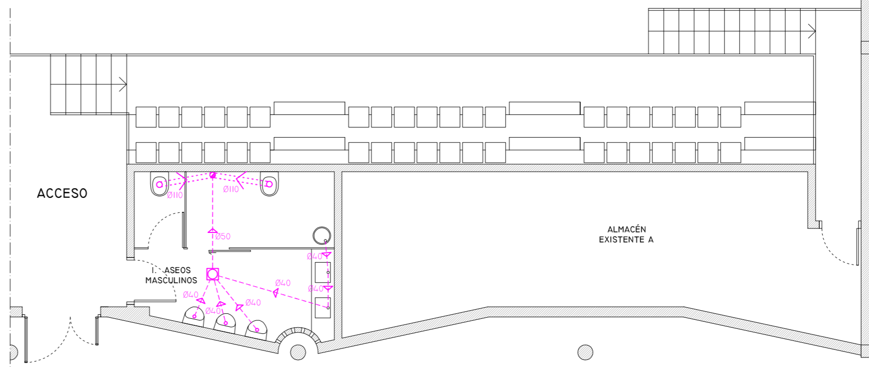
PLANTA ASEOS - LATERAL A - INSTALACIÓN DE FONTANERÍA 1/75
