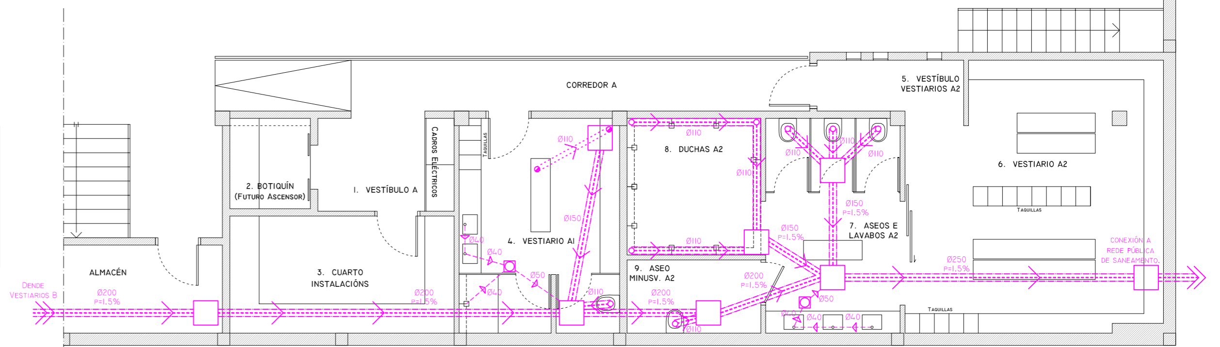
PLANTA VESTIARIOS - LATERAL A - INSTALACIÓN DE FONTANERÍA 1/75
