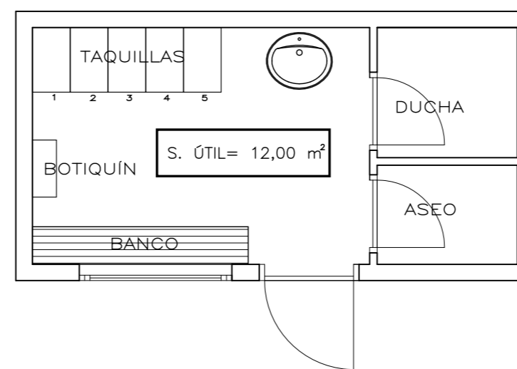
PLANTA DE CASETA DE VESTUARIOS. E:1/50
