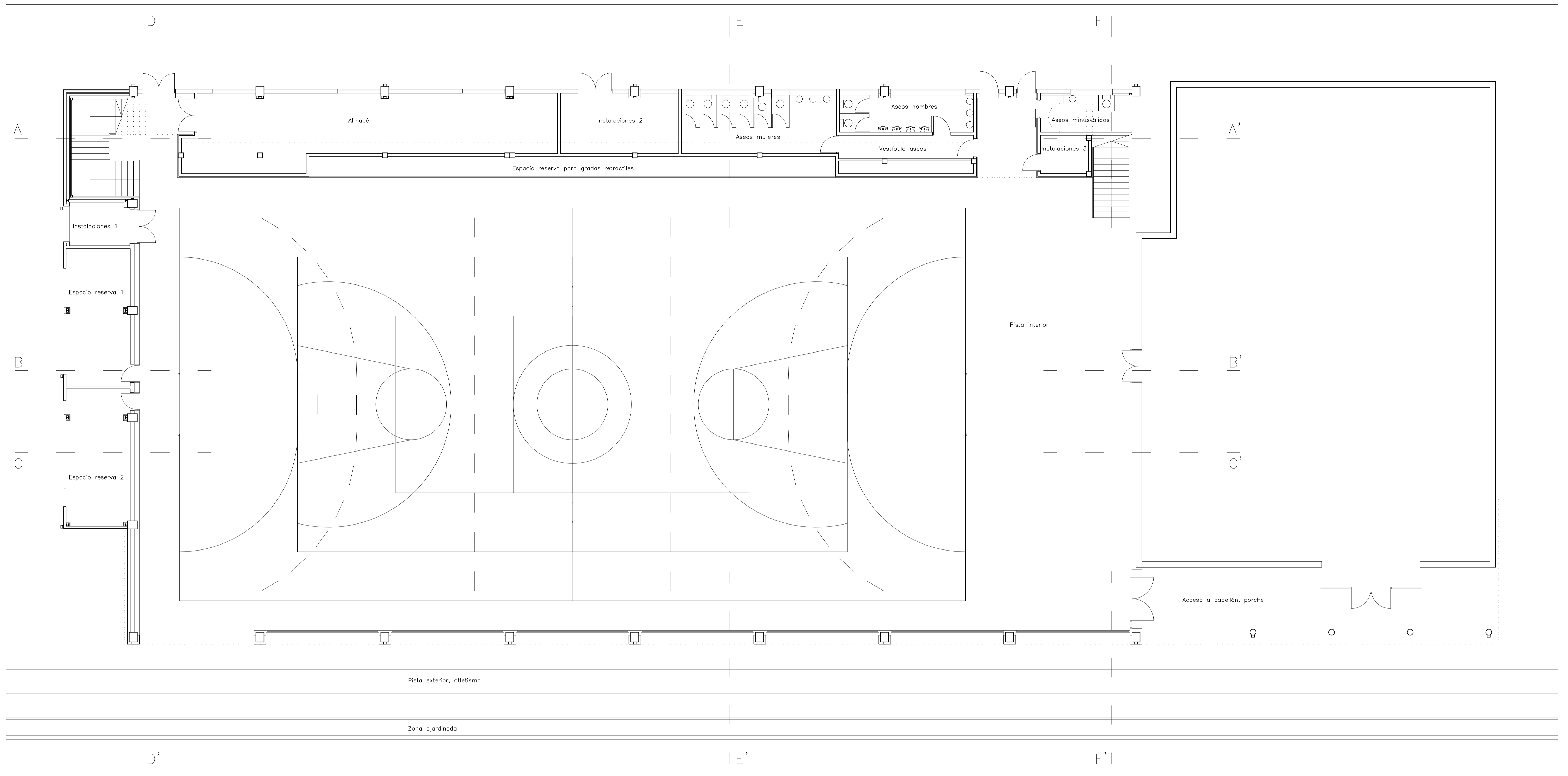
Planta baja. Estado reformado
