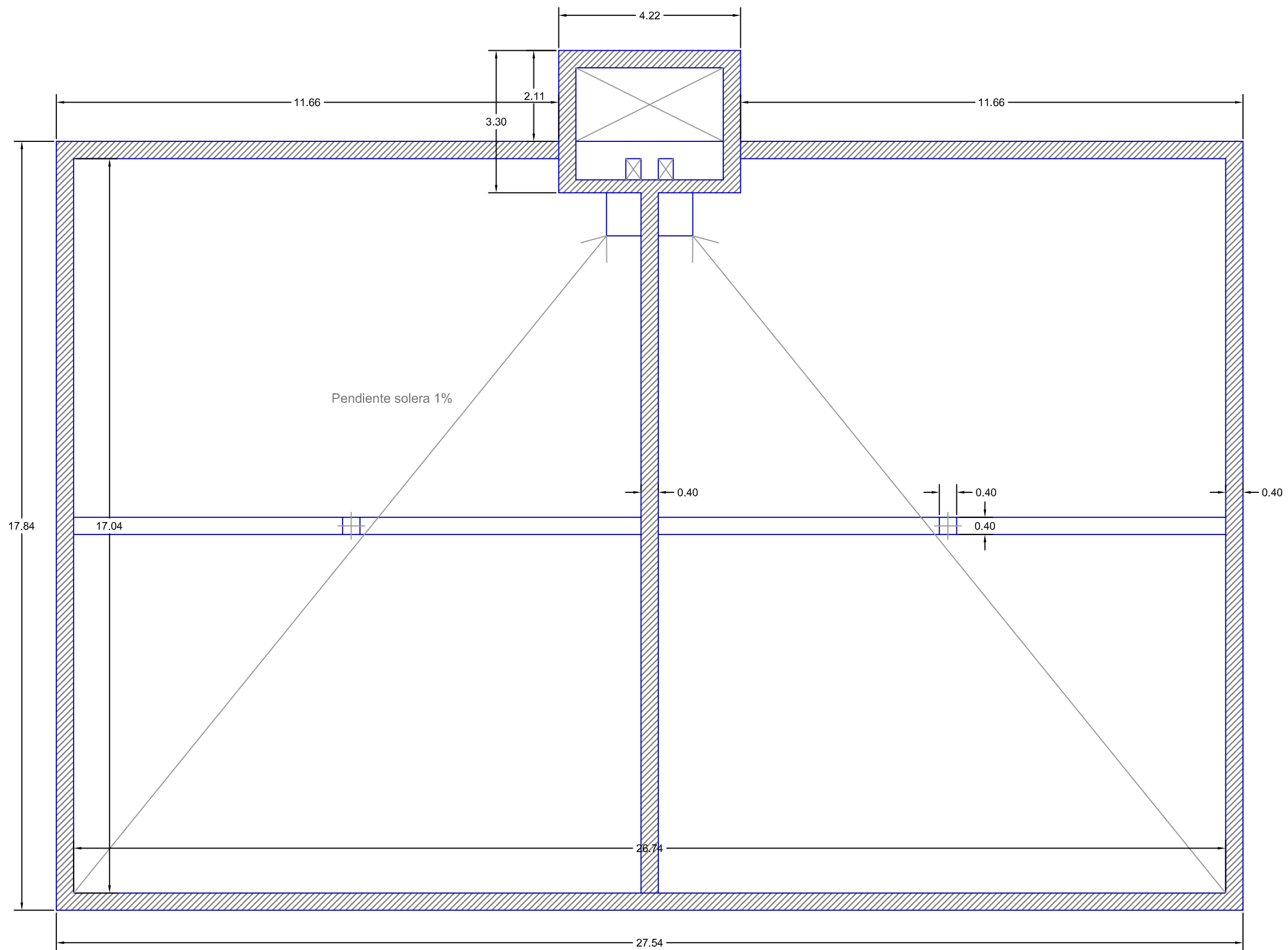
Planta depósito
