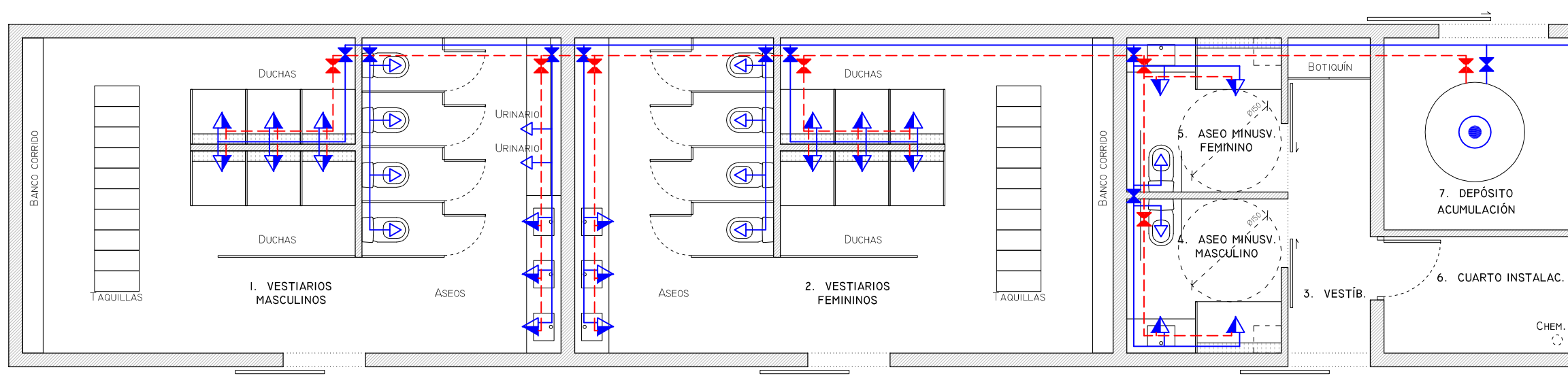
ESQUEMA DA INSTALACIÓN DE FONTANERÍA 1/75
