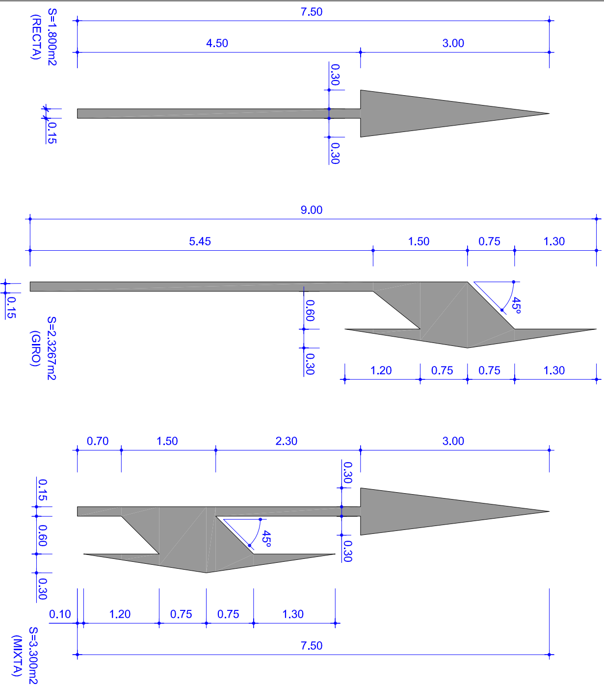
M-5.1 VIA CON VM > 60Km/h
