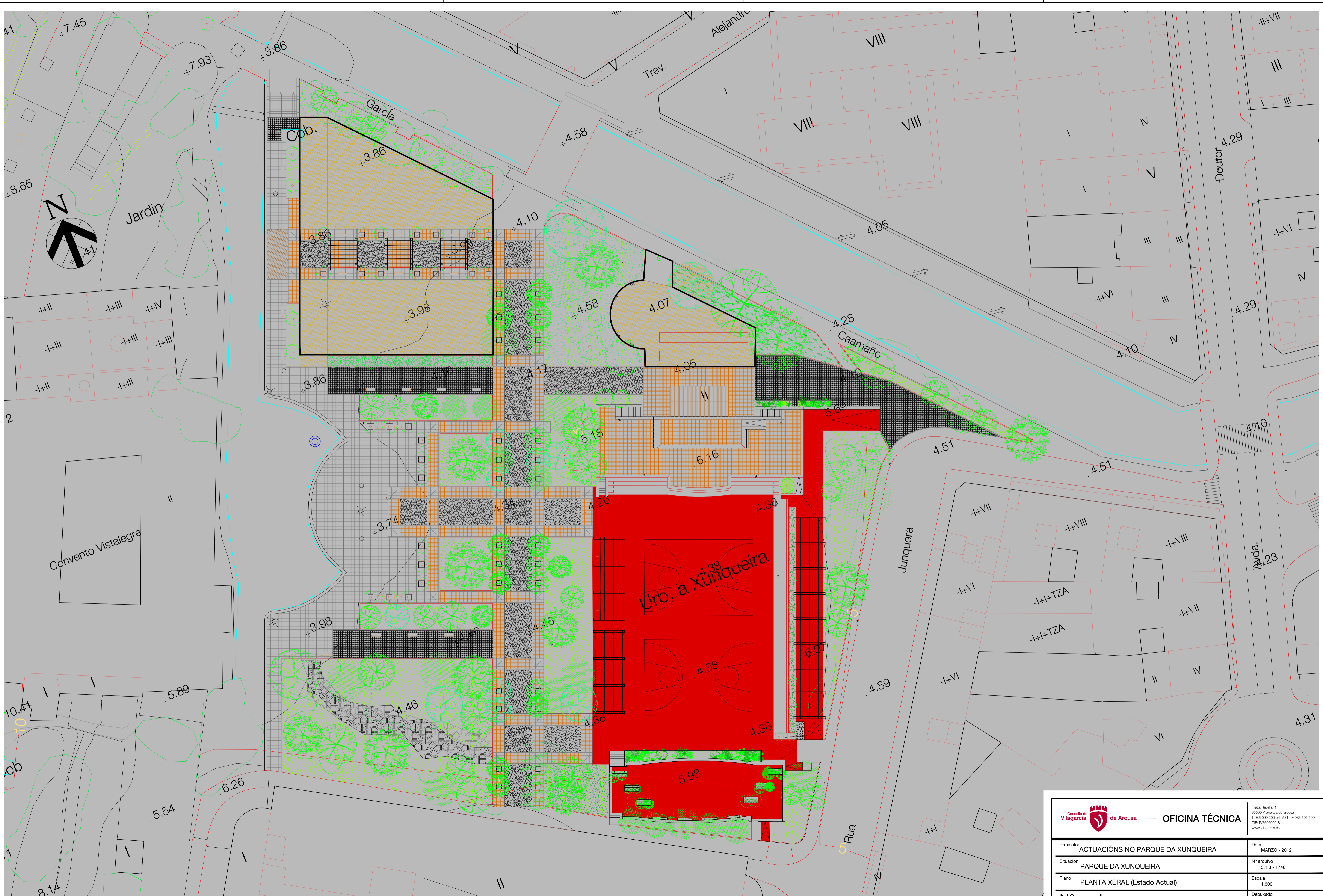
PLANTA XERAL - ESTADO ACTUAL ESCALA 1:300
