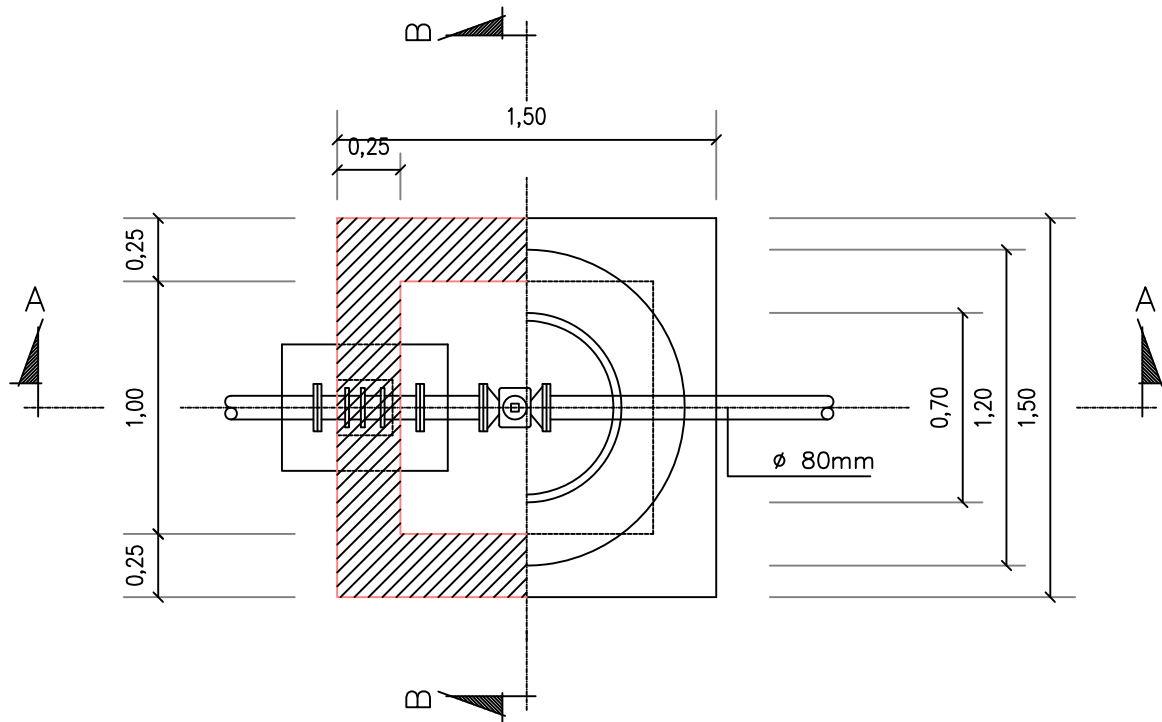
PLANTA – SECCION
