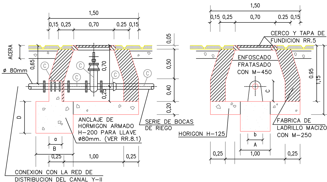
SECCION A-A
