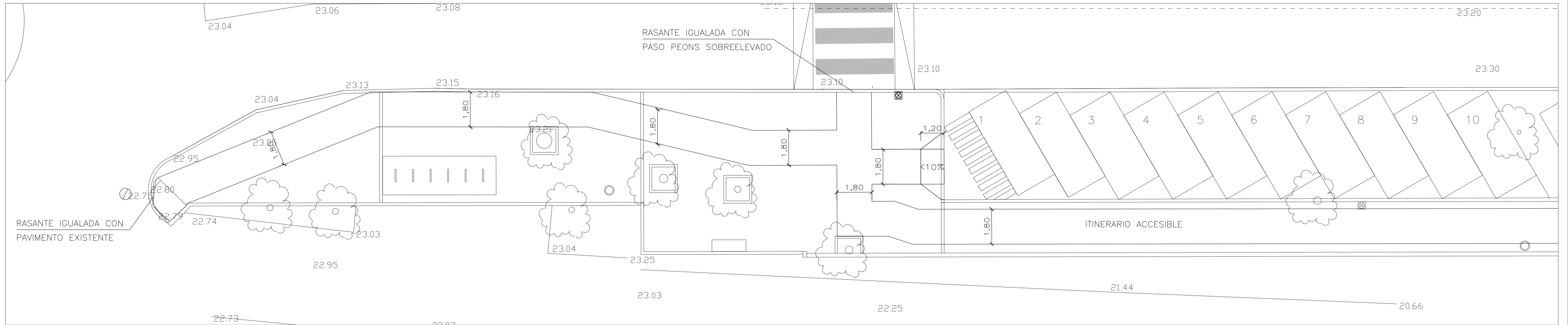
XUSTIFICACION ACCESIBILIDADE ZONA 1. E 1/100
