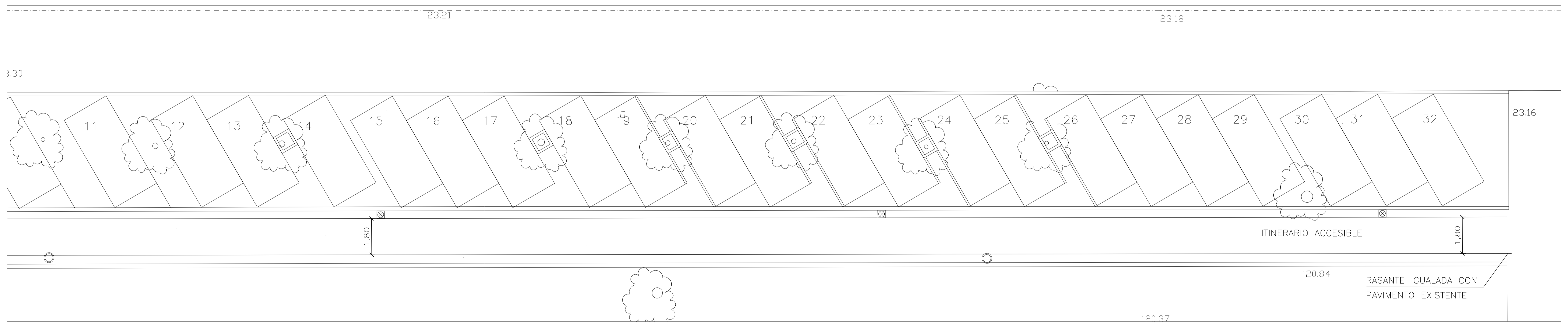
XUSTIFICACION ACCESIBILIDADE ZONA 2. E 1/100
