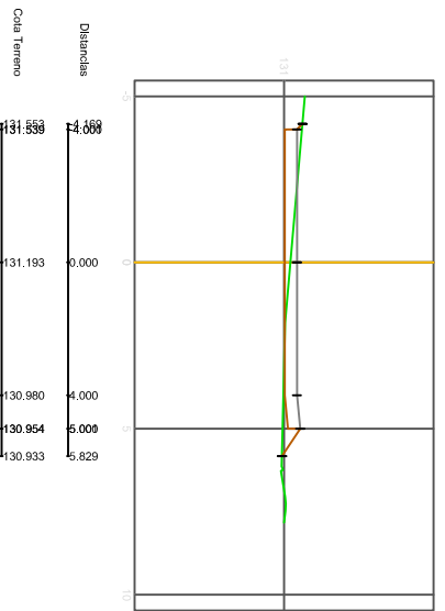
Z=131.193 Z=131.365 Z=131.015 SH=0.343 SH=1.603 SH=0.000 SH= 3.330 P.K.=1040.000 - Perfil N. 5
